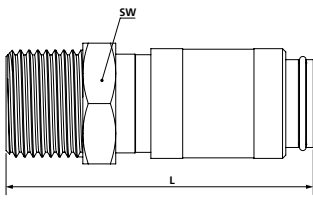
Kupplung mit Außengewinde
