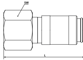
Kupplung mit Innengewinde
