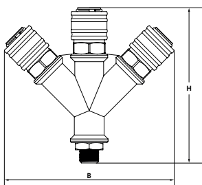
Verteiler mit 3 Schnellverschlusskupplungen, Außengewinde
